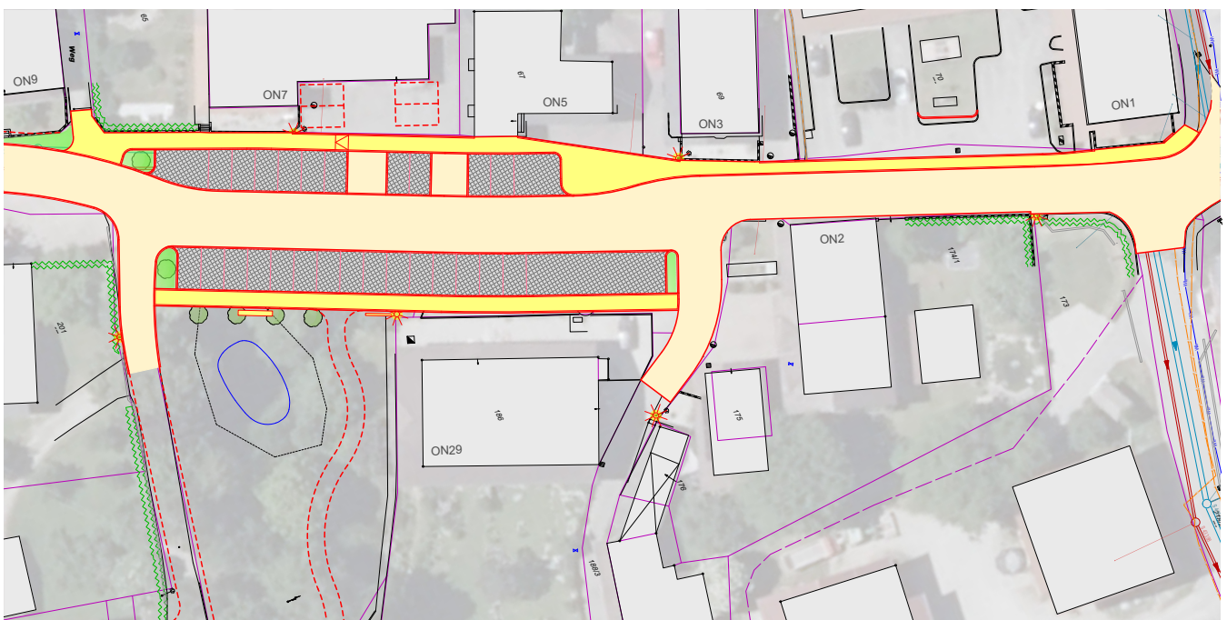
Plan der Sanierung Dorfstraße und Dorfplatz.
